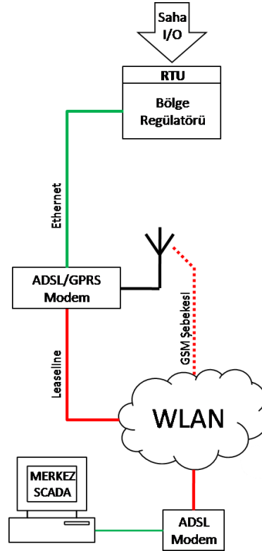
Şekil 2: Bölge Regülatörü RTU Bağlantıları ve Haberleşmesi
