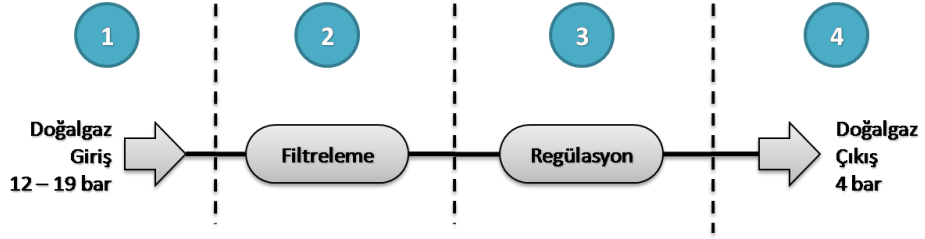
Şekil 1: Bölge Regülatörü Proses Şeması
