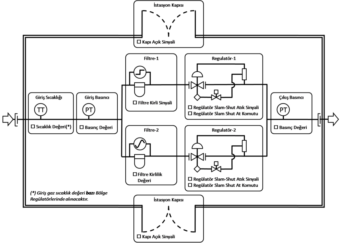
Şekil 3: Bölge Regülatörü
